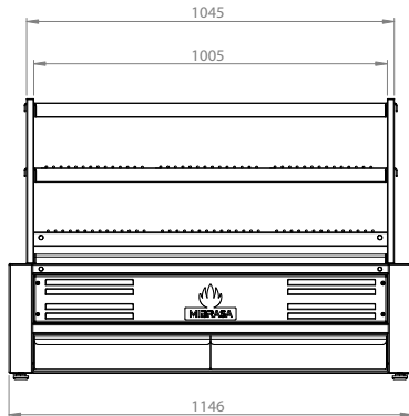
Vue frontale
