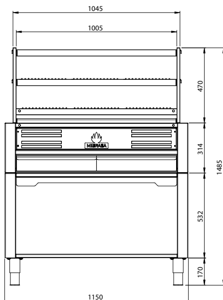
VUE FRONTALE
