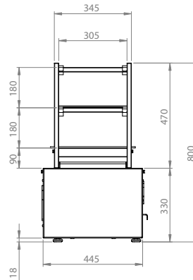
Vue latérale
