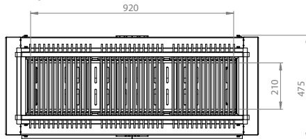
Vue supérieure
