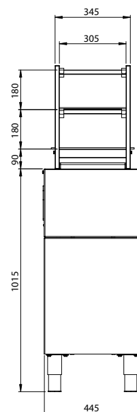
VUE LATÉRALE
