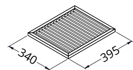
DIMENSIONES DEL SOPORTE BANDEJA
