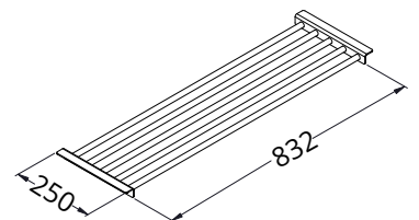
DIMENSIONS DEL SUPORT DE COCCIÓ VERTICAL
