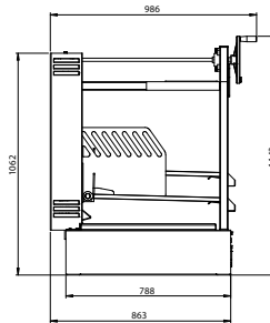
Quemador
