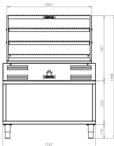
VUE FRONTAL
