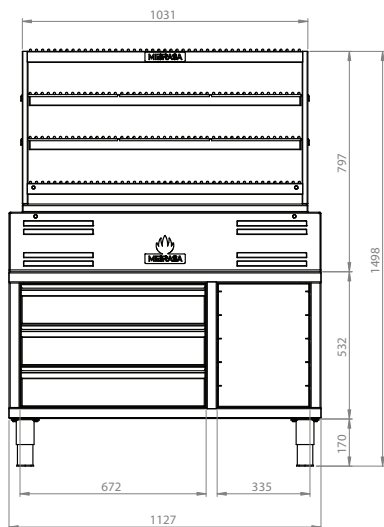
VUE FRONTAL
