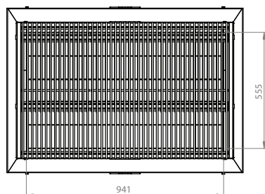
VUE SUPÉRIEURE
