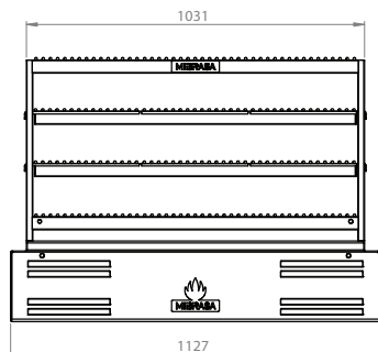
VUE FRONTAL
