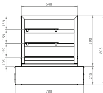
VUE LATÉRALE
